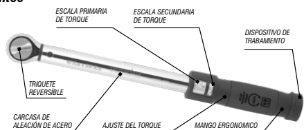
Figura 1 – Componentes de los modelos con encaje 1/2"
