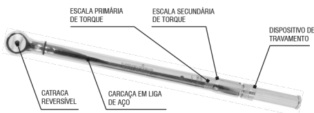
Figura 2 – Componentes modelos com encaixe 3/4"
