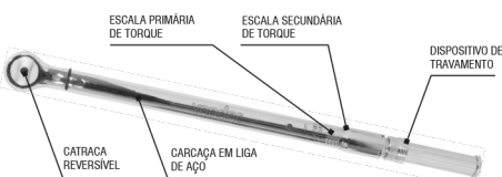
Figura 2 – Componentes de los modelos con encaje 3/4"
